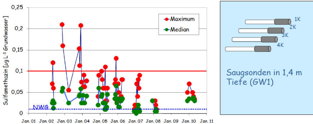
Abbildung 32: Sulfadimidin-Konzentrationen an der BDF in Dinklage in 1,4 m Tiefe (links) sowie Einbau der 4 Saugsonden in den Boden (rechts, Höper 2011)
