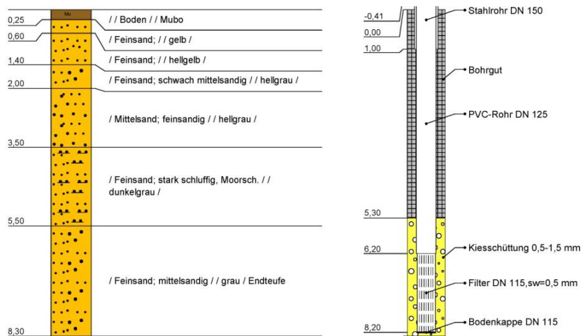
Abbildung 34: Schichtenverzeichnis der Messstelle Dwertge (zur Verfügung gestellt vom NLWKN)
