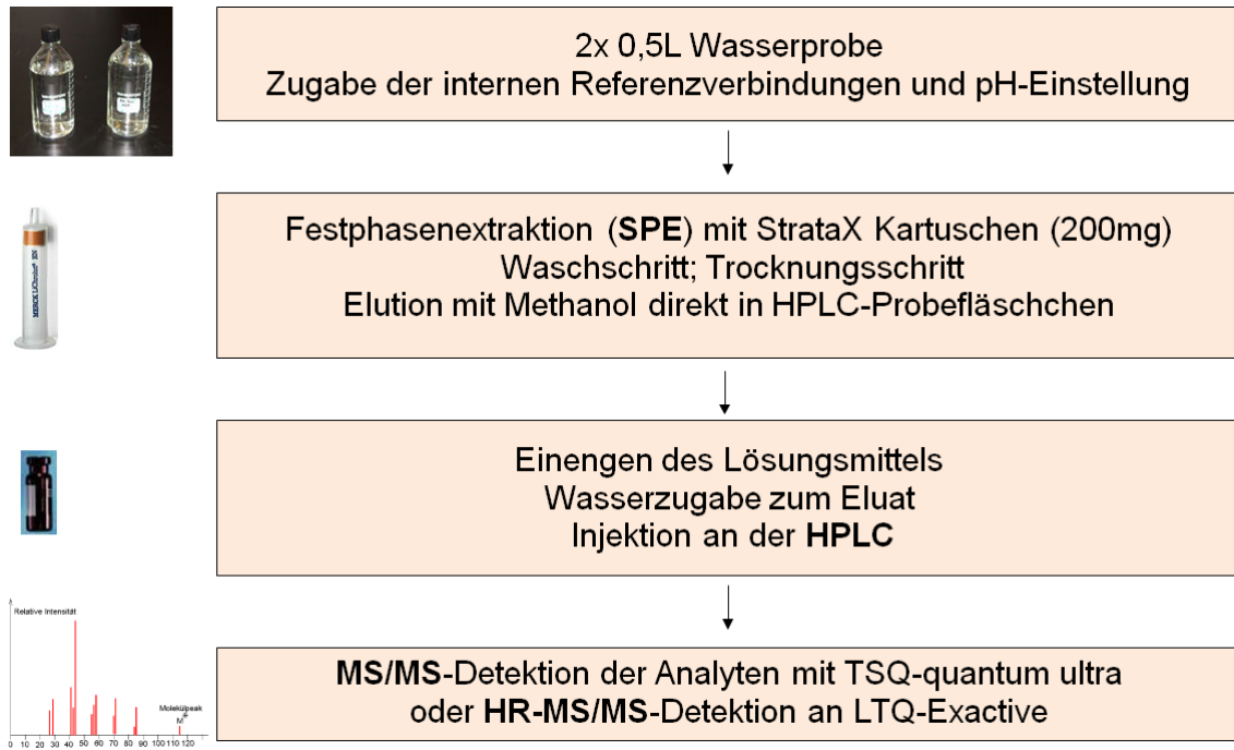
Abbildung 7: Übersicht über die durchgeführte Probenvorbereitung, Trennung und Detektion am Beispiel der Sulfonamide
