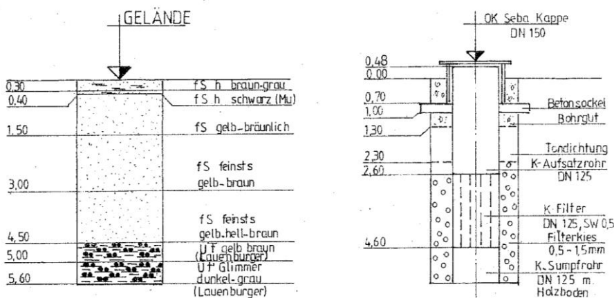
Abbildung 67: Schichtenverzeichnis (links) und Ausbau (rechts) der Messstelle Bösel I des NLWKN (zur Verfügung gestellt von der Betriebsstelle Cloppenburg des NLWKN)
