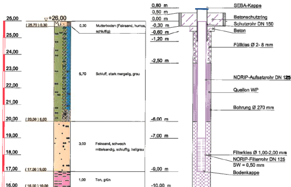
Abbildung 30: Schichtenverzeichnis der Messstelle Itterbeck I in Niedersachsen (zur Verfügung gestellt vom NLWKN)
