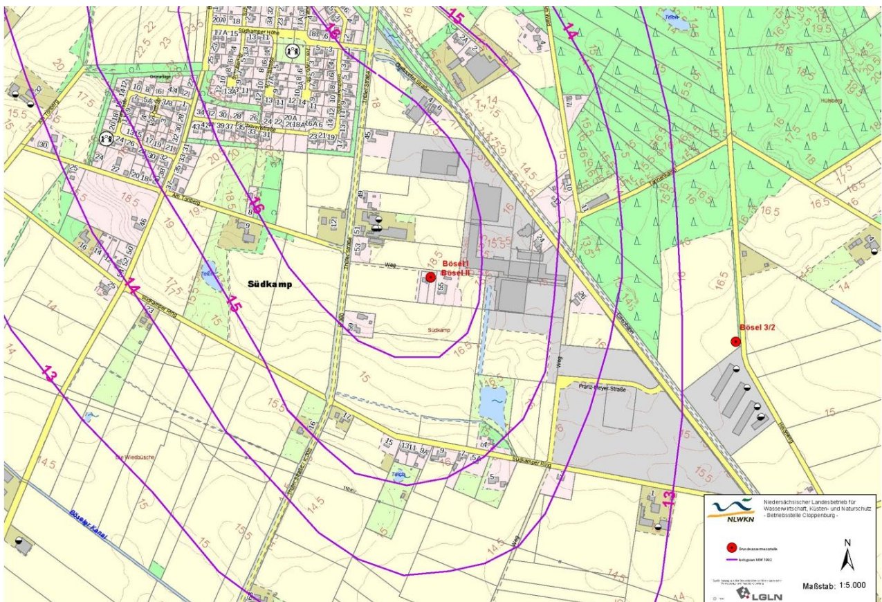
Abbildung 66: Lageplan der Messstelle Bösel I mit Informationen des NLWKN zum Umfeld des Messstellenstandortes (frdl. zur Verfügung gestellt vom NLWKN, Betriebsstelle Cloppenburg)
