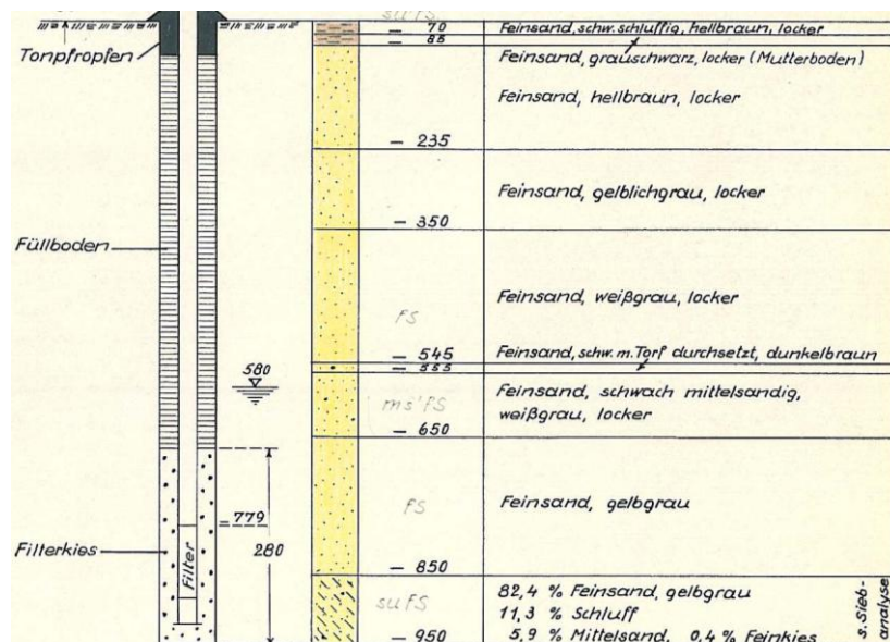
Abbildung 34: Schichtenverzeichnis der Messstelle Dwertge (zur Verfügung gestellt vom NLWKN)
